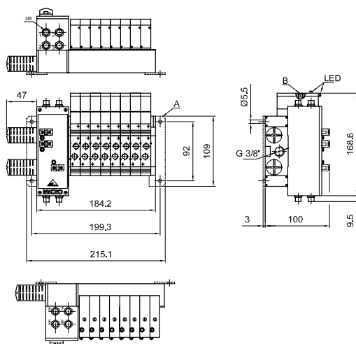
AS-i duplo solenóide VM15-B (8I / 8O)
