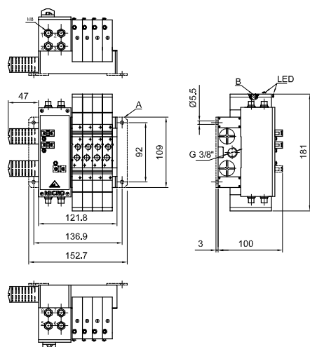
AS-i duplo solenóide VM15-B (8I / 8O)
