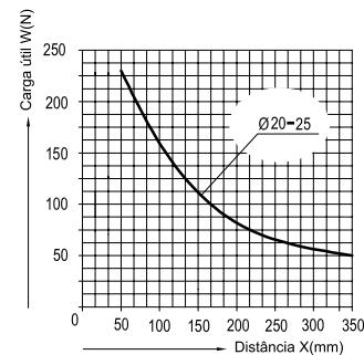
Gráfico da carga útil (W) em Newton versus a distância (X) em milímetros para o tubo Ø20-25. A curva mostra uma diminuição da carga útil com o aumento da distância, partindo de aproximadamente 145 N a 50 mm até cerca de 45 N a 250 mm.
