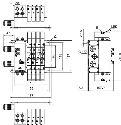
AS-i duplo solenóide VM18-B (8I / 8O)
