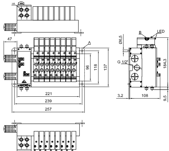
AS-i duplo solenóide VM18-B (8I / 8O)
