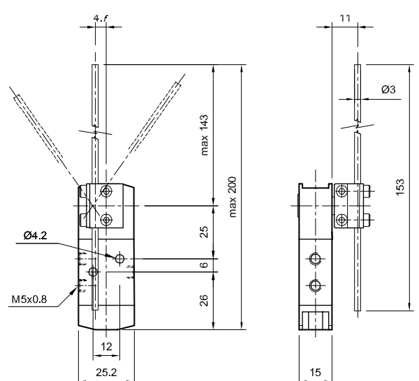
Comando por vareta lateral regulável bidirec.
