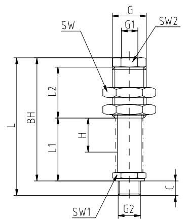
FSTE-1/8 ... FSTE-1/4 (-VG)
