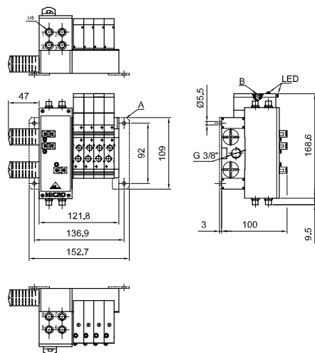
AS-i simples solenóide VM15-B (8I / 8O)
