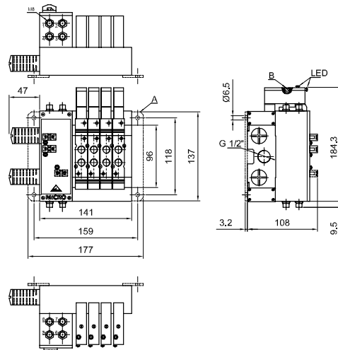
AS-i simples solenóide VM18-B (8I / 8O)
